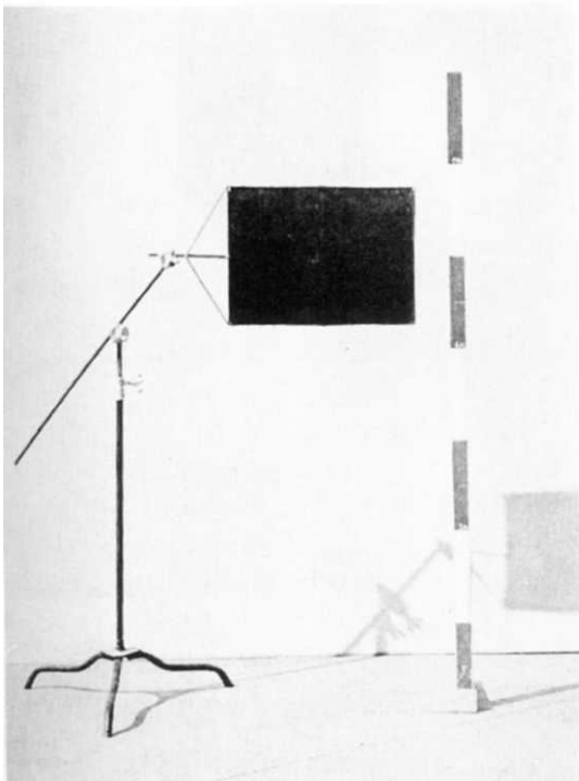
Fig. 17 Flag
