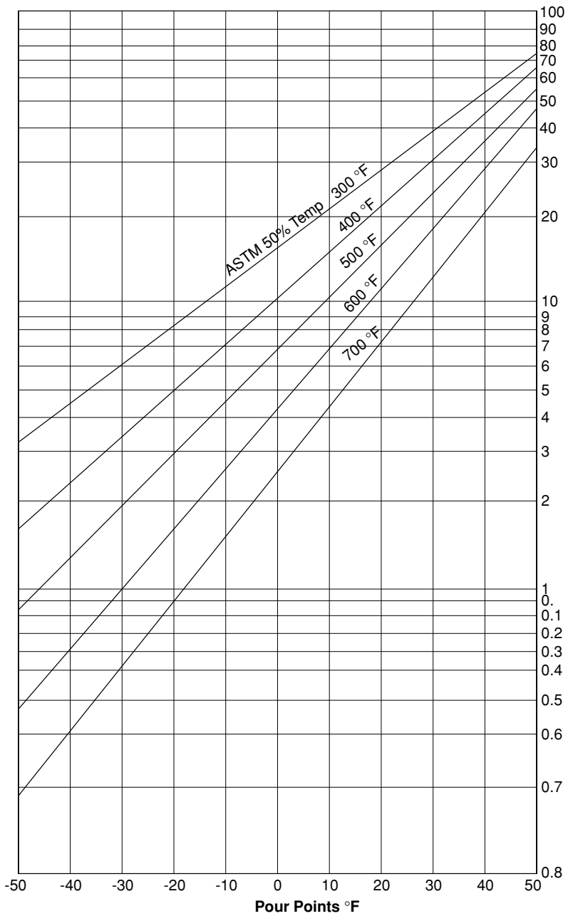
Figure 1.12. Pour point blending index.
