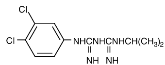
Chlorproguanil
