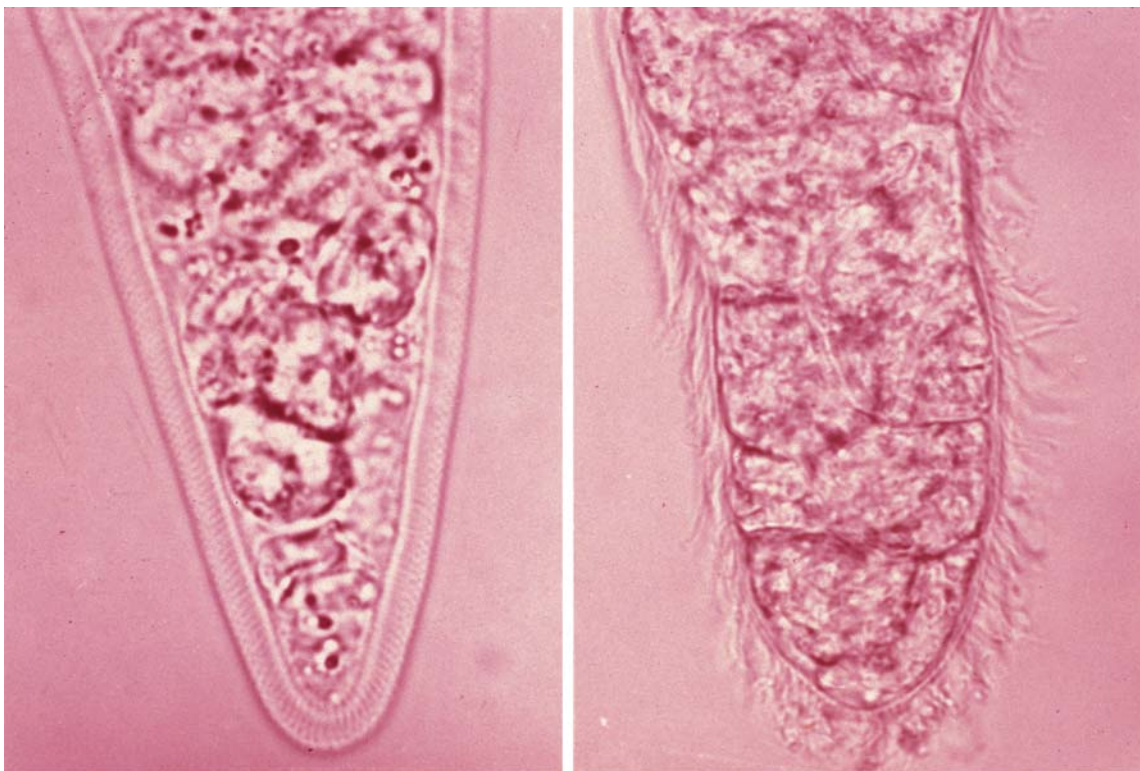
S. ovicanis
