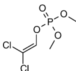
dichlorvos (DDVP)
