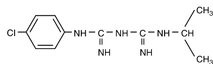
Proguanil
