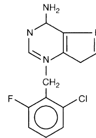
Arprinocid
