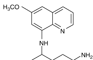
(Primaquine)
