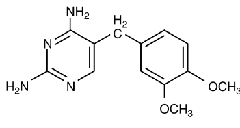
Diaveridine
