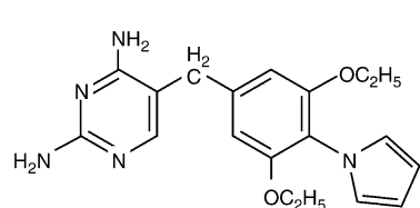
Epiroprim
