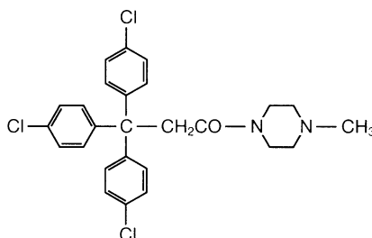
Hetolin
