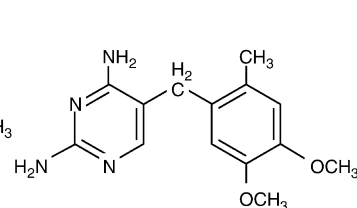
Ormethoprim
