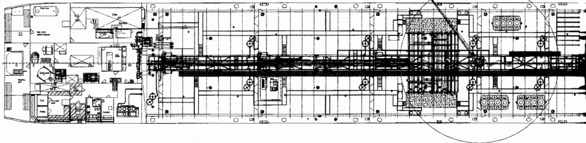
Tweendeck
