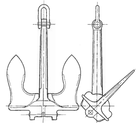
Baldt anchor
